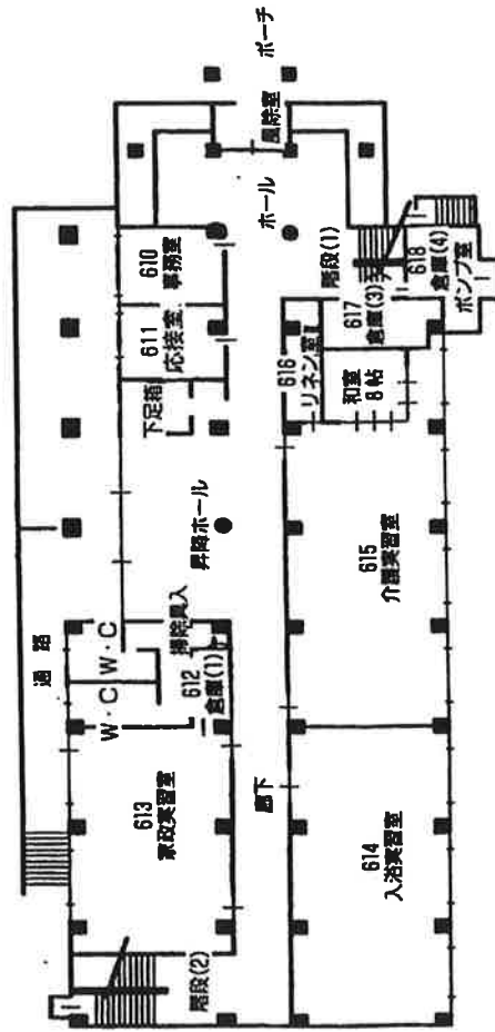
一階平面図
