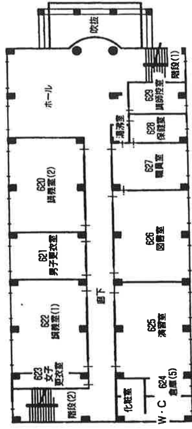
二階平面図
